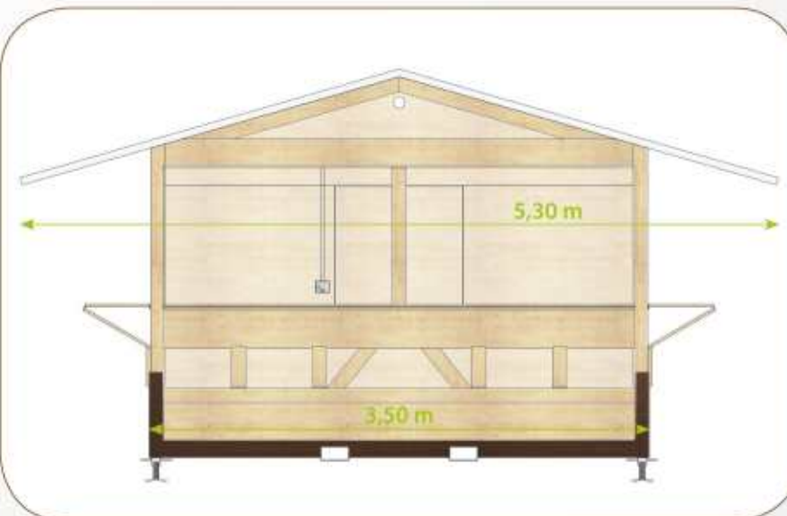
VISTA FRONTALE VORDERANSICHT FRONT VIEW
