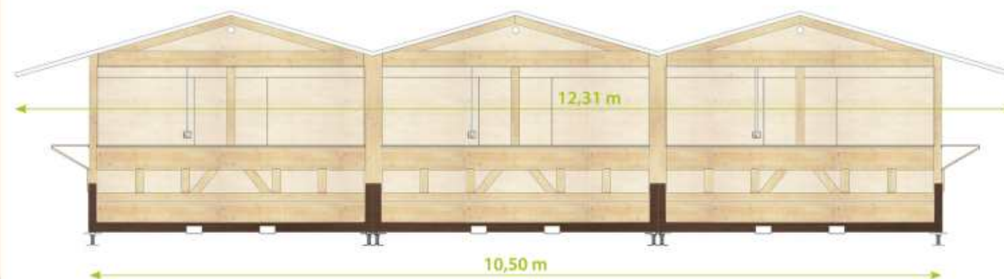
VISTA FRONTALE VORDERANSICHT FRONT VIEW
