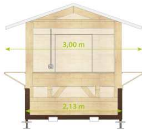
VISTA FRONTALE VORDERANSICHT FRONT VIEW
