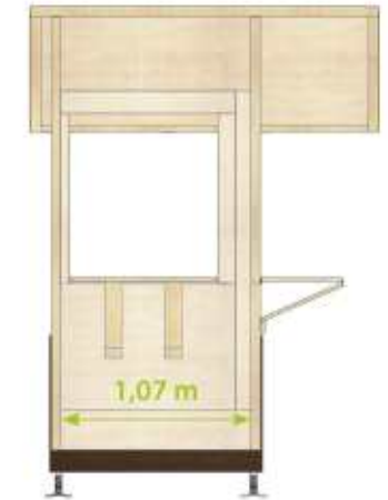
VISTA INTERNO LATO SINISTRO LINKE SEITENANSICHT INNEN INTERIOR VIEW LEFT SIDE
