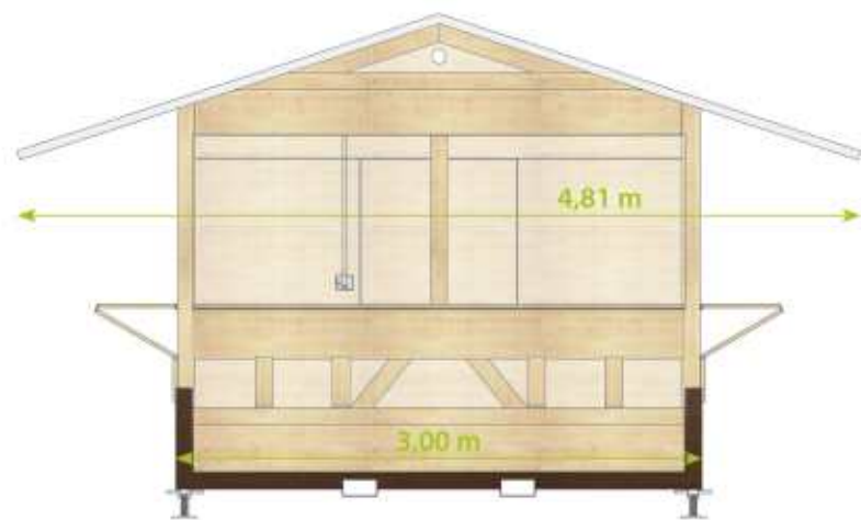
VISTA FRONTALE VORDERANSICHT FRONT VIEW
