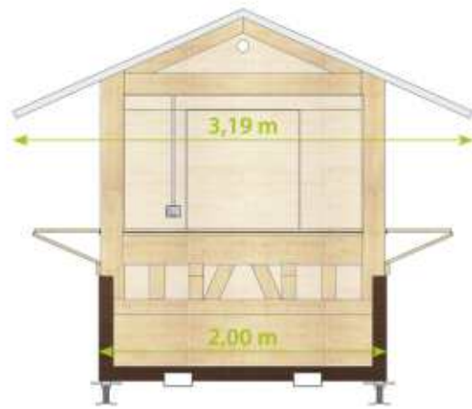
VISTA FRONTALE VORDERANSICHT FRONT VIEW
