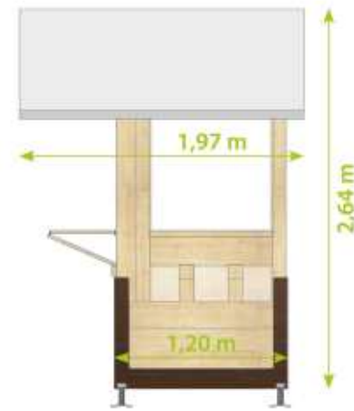
VISTA LATO DESTRO RECHTE SEITENANSICHT RIGHT SIDE VIEW
