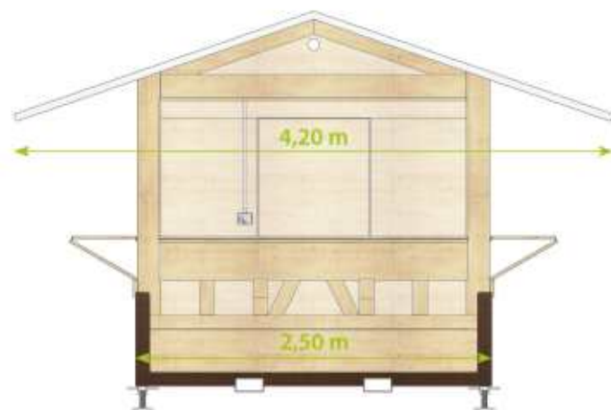
VISTA FRONTALE VORDERANSICHT FRONT VIEW
